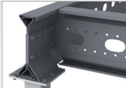
Hauptträger
