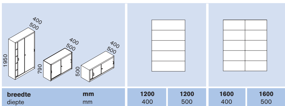
Schuifdeurkast, hoogte 1950 mm, met 4 legborden
