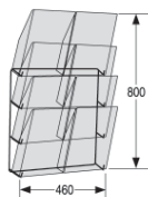
5. wandopstelling 2 × 4 B 460 × D 190 × H 800 mm
