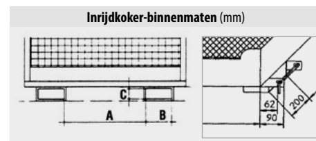
Veiligheidsbouten beschermen tegen onbedoeld afglijden
